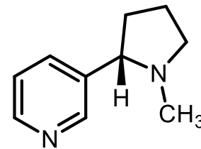
Nicotin (Pyridinalkaloid)
